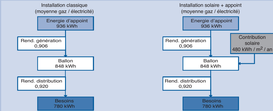
Figure 33. : Contribution solaire et énergie d'appoint pour l'ECS
