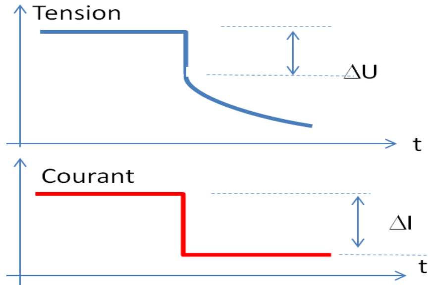
Mesure de résistance à 1 seconde
