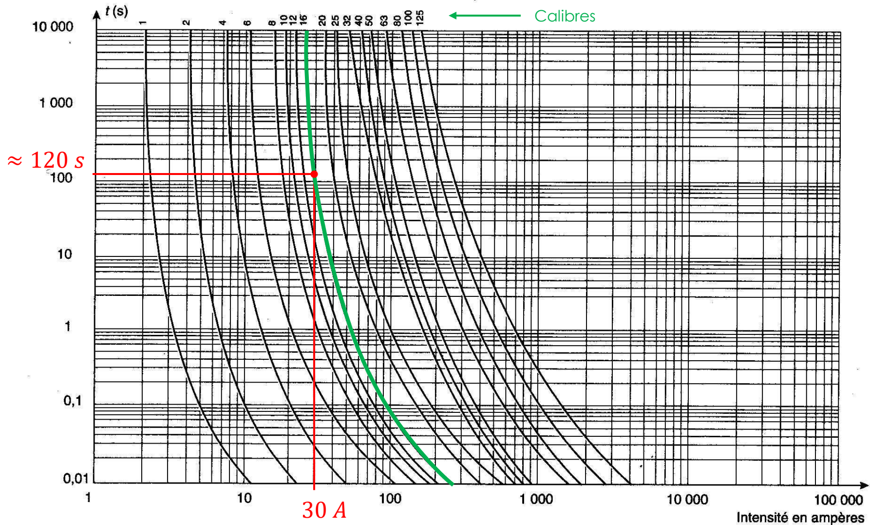
Courbes de fusion des cartouches type gG.
