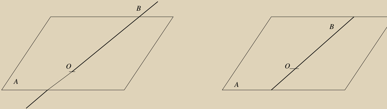
FIGURE C.1.1 – plan et droite
